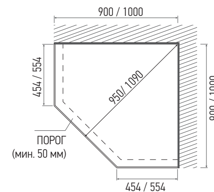
СХЕМА ПОДИУМА
