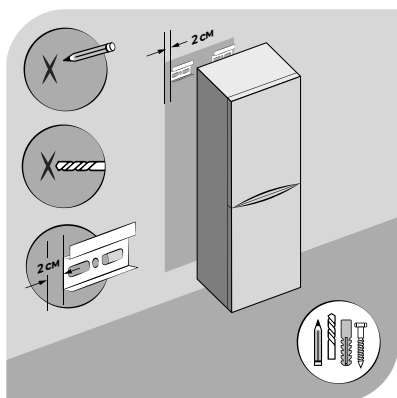
Установка шкафа
