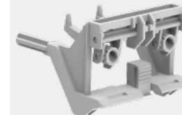
Блок рычагов с механическим управлением
